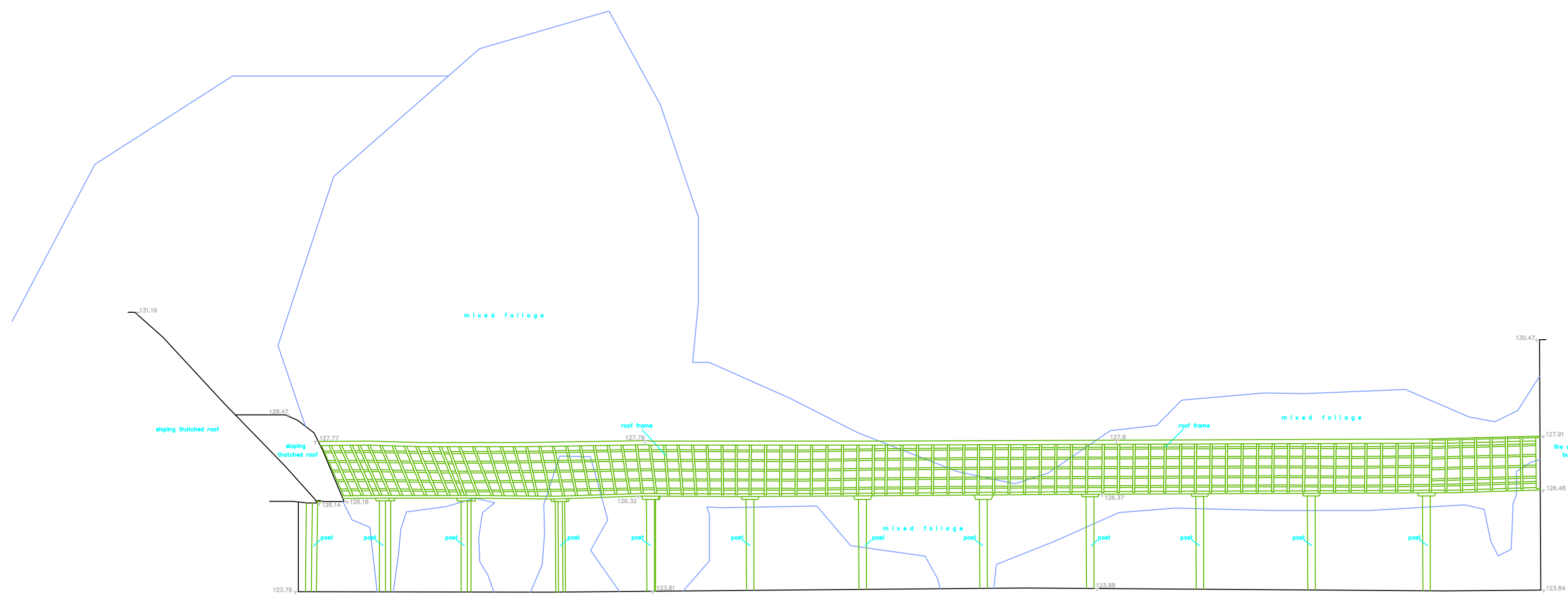
ELEVATION E
