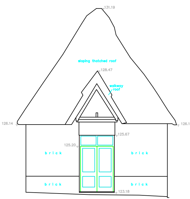
ELEVATION B
