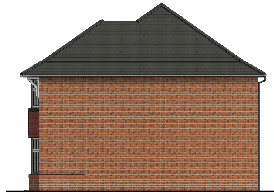
Right Elevation
