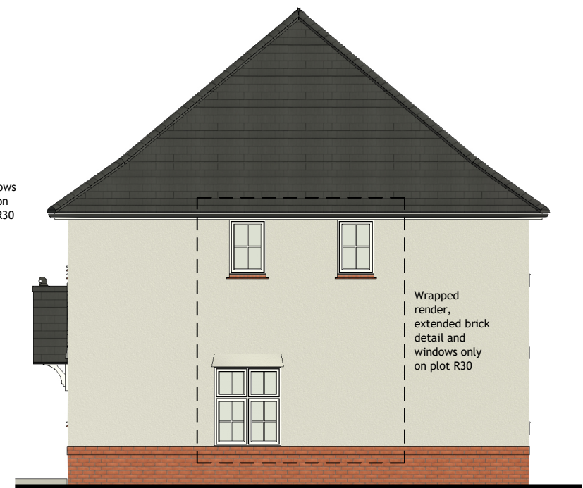
Right Elevation
