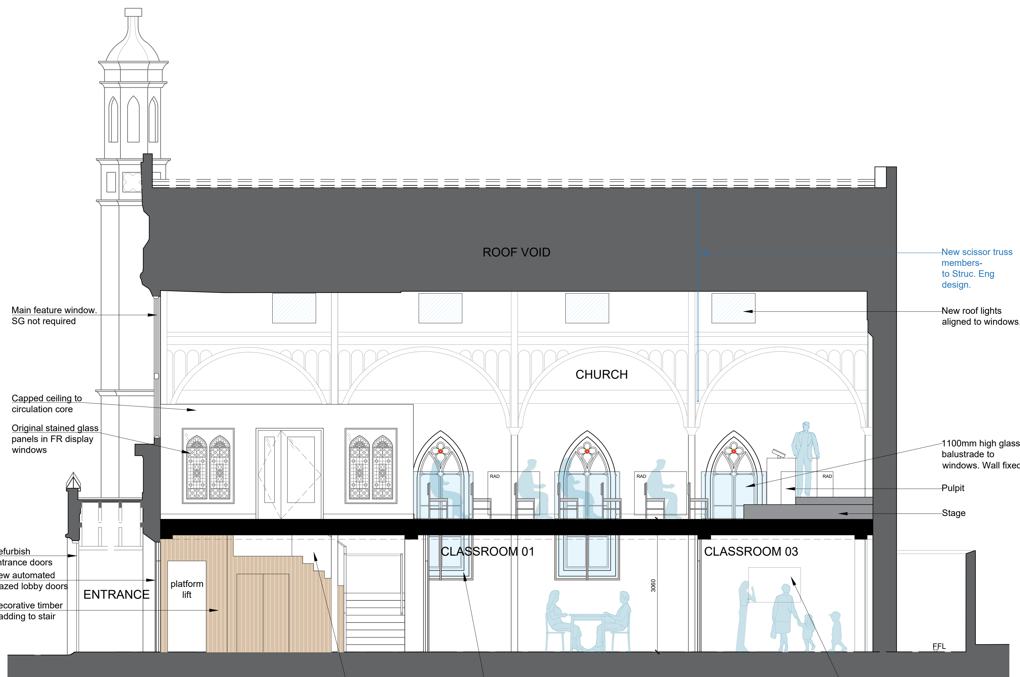
SECTION D-D
