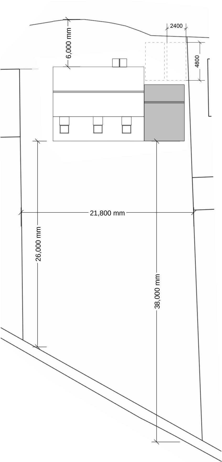
SITE PLAN 1:250
