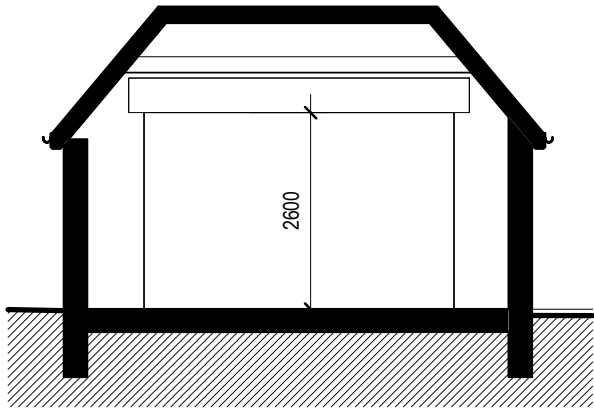
Section A-A 1 : 100
