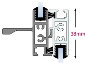
Box interlock
